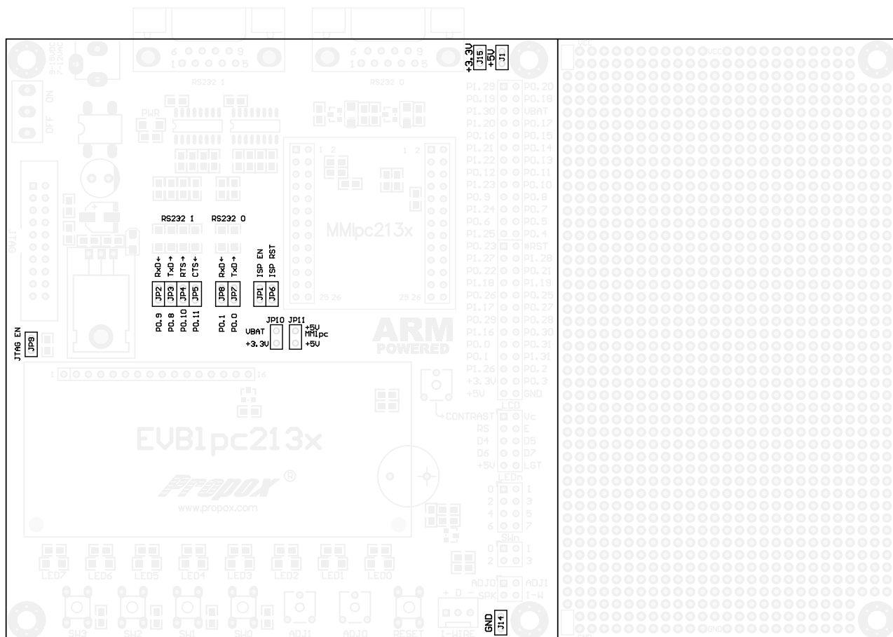
Rysunek 2 Rozmieszczenie zworek konfiguracyjnych na płycie.
