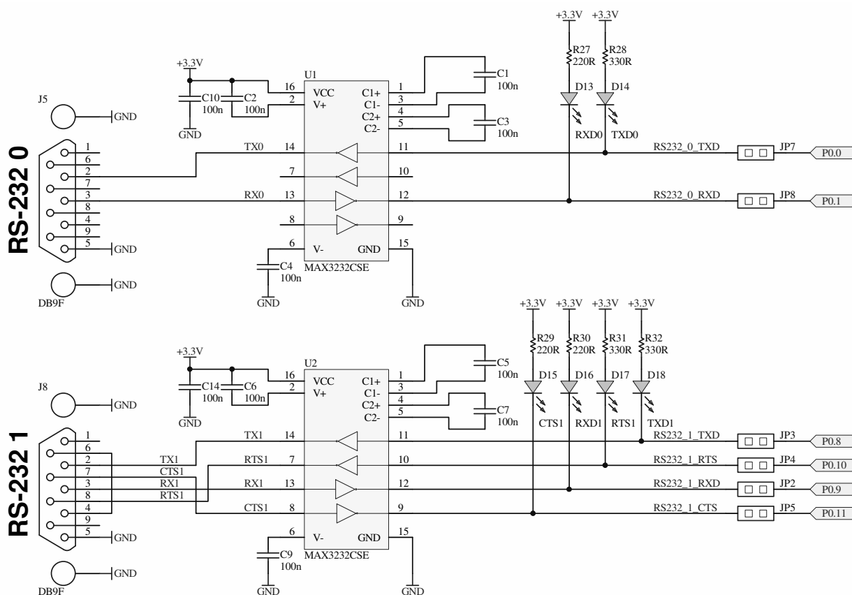
Rysunek 11 Podłączenie portu RS-232 do MMlpc213x.
