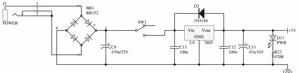
Rysunek 3 Implementacja zasilacza na płycie EVBlpc213x.
