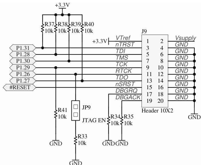
Rysunek 14 Podłączenie złącza JTAG na płycie EVBlpc213x.
