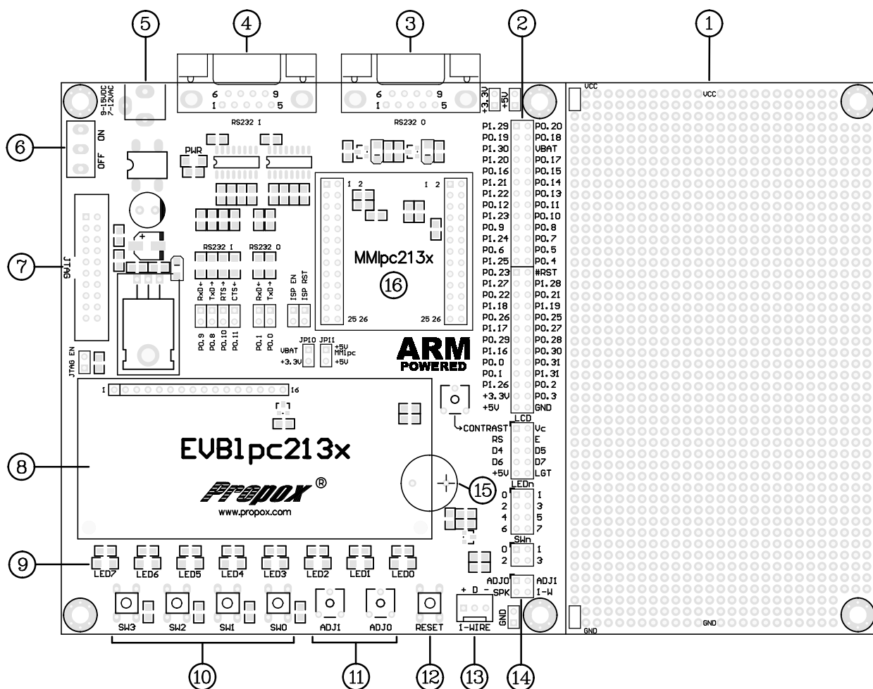
Rysunek 1 Rozmieszczenie elementów na płycie EVB1pc213x.
