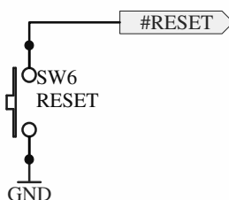
Rysunek 10 Implementacja przycisku RESET.
