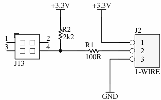
Rysunek 12 Podłączenie złącza 1-Wire.
