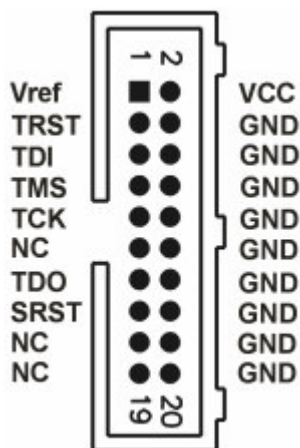
Rysunek 13 Złącze JTAG.
